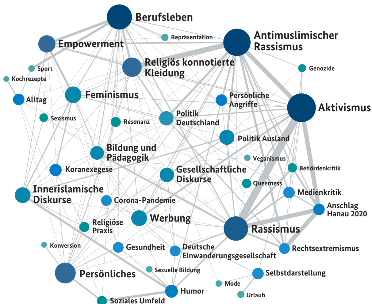
Abbildung 7.5: Thematische Netzwerkanalyse
